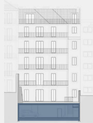
Alçado tardoz
